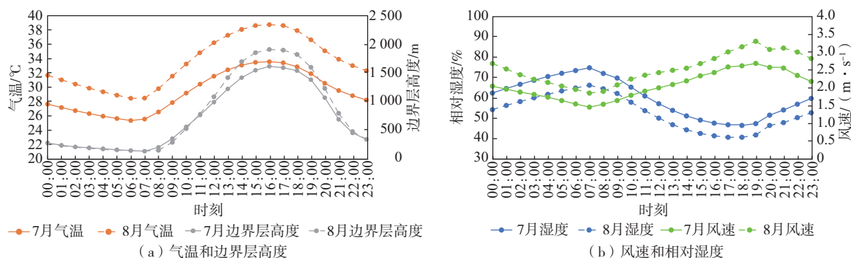
图5 7、8月重庆气象条件日变化
