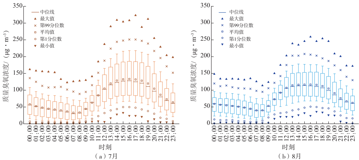
图4 7、8月重庆臭氧日变化箱线图
