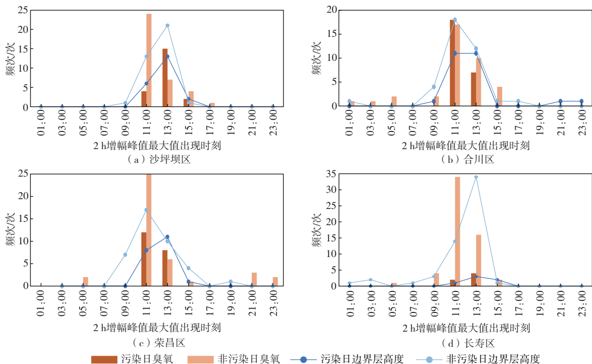
图8 4个代表县(区)在2022年7—8月的污染日和非污染日中臭氧质量浓度、边界层高度2 h增幅最大值出现时间频次分布
