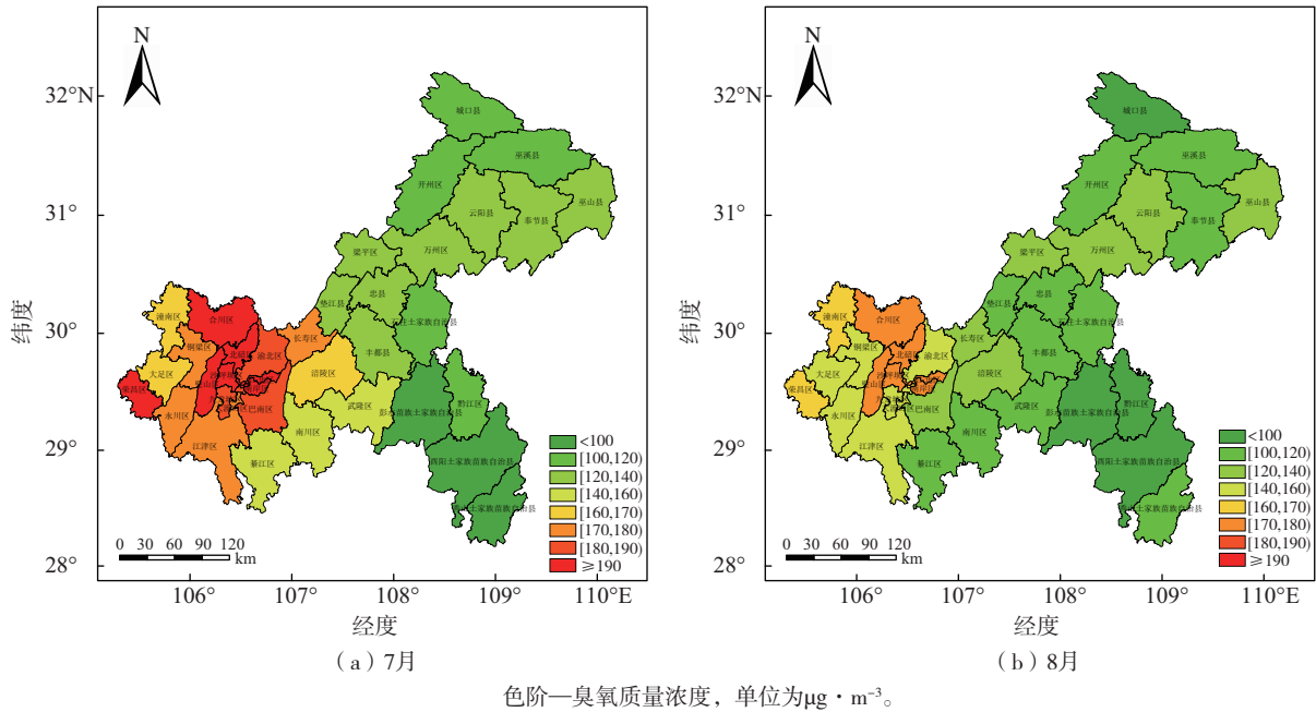
图3 7、8月重庆MDA8-O 3 第90分位数空间分布
