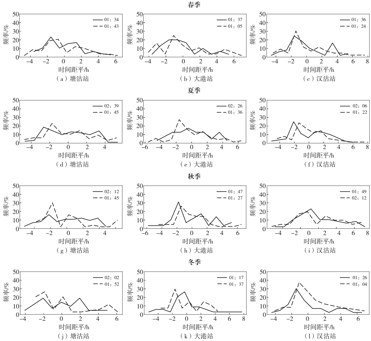
实线—ERA5数据;虚线—站点数据;图例中时间—平均结束时间。
