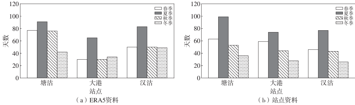
图 5 不同季节各站海陆风日数对比
