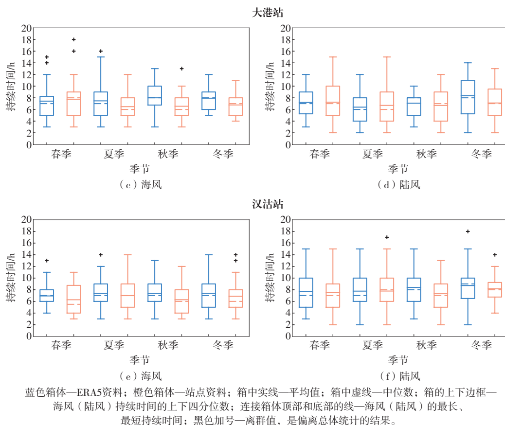
图 10 各站点各季节海风、陆风持续时间对比
