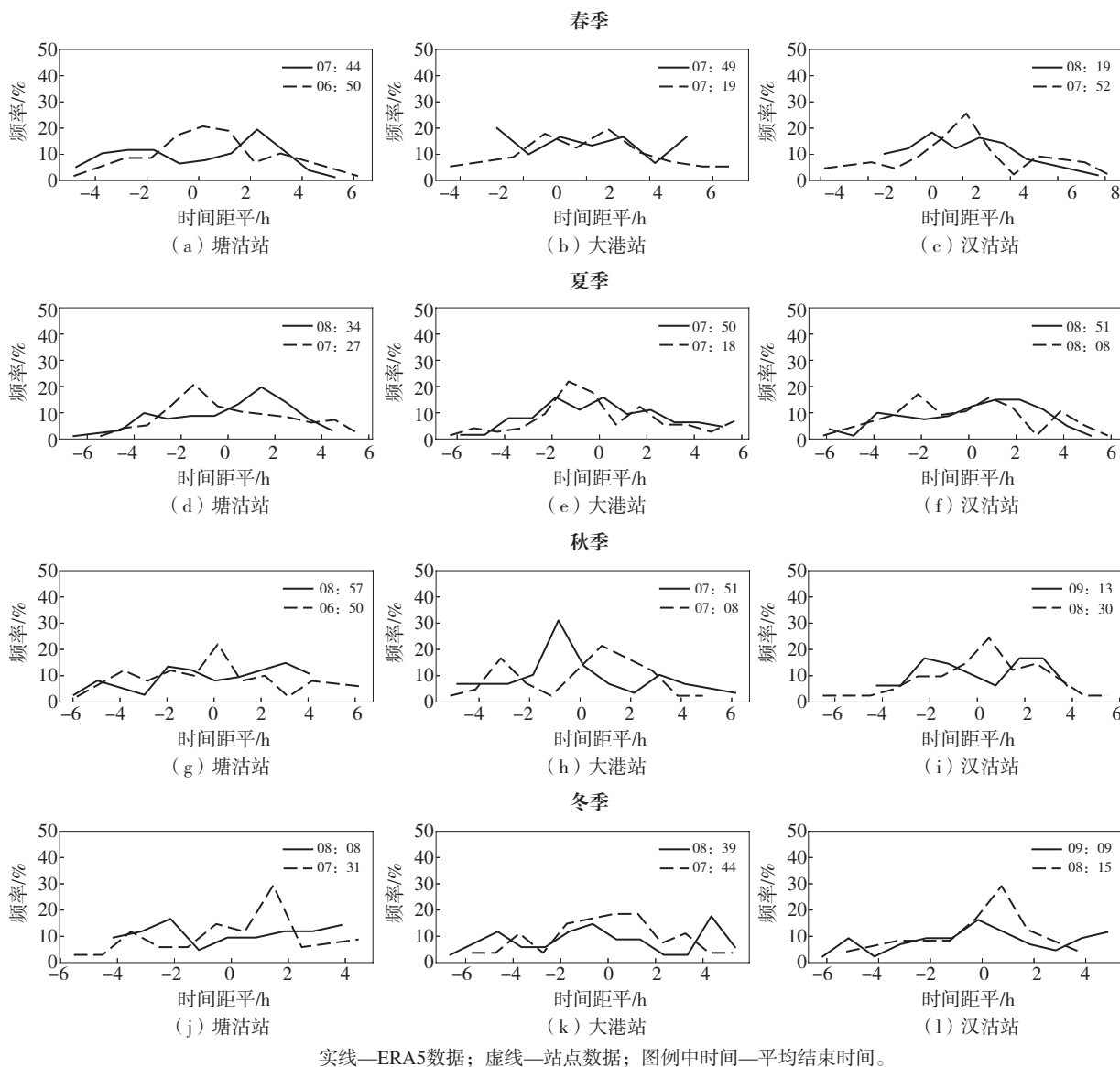
图9 不同季节陆风结束时间距平分布
