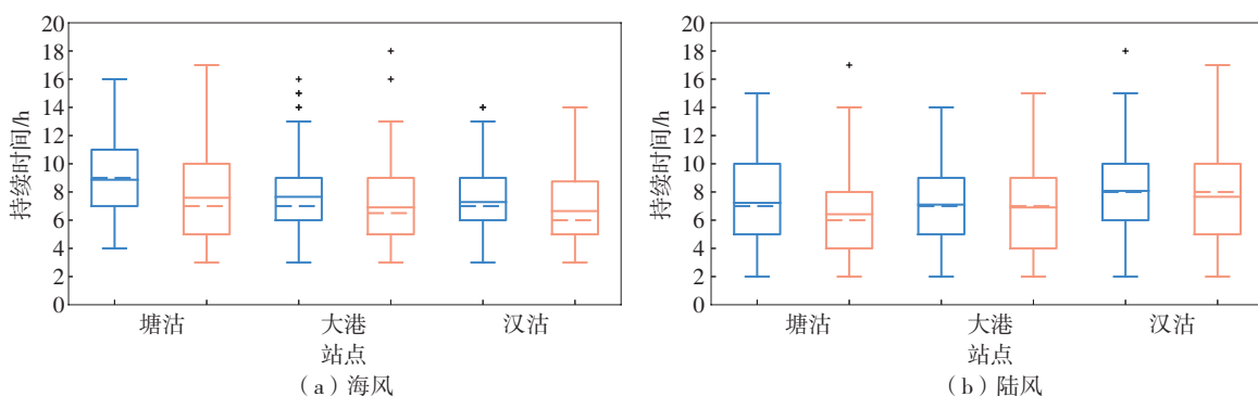
蓝色箱体—ERA5资料；橙色箱体—站点资料；箱中实线—平均值；箱中虚线—中位数；箱的上下边框—海风（陆风）持续时间的上下四分位数；连接箱体顶部和底部的线—海风（陆风）的最长、最短持续时间；黑色加号—离群值，是偏离总体统计的结果。
