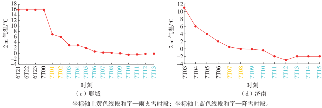
图 6 925 hPa、1 000 hPa 以及 2 m 气温逐时分布 Fig.6 Hourly distribution of temperature at 925 hPa, 1 000 hPa, and 2 m
