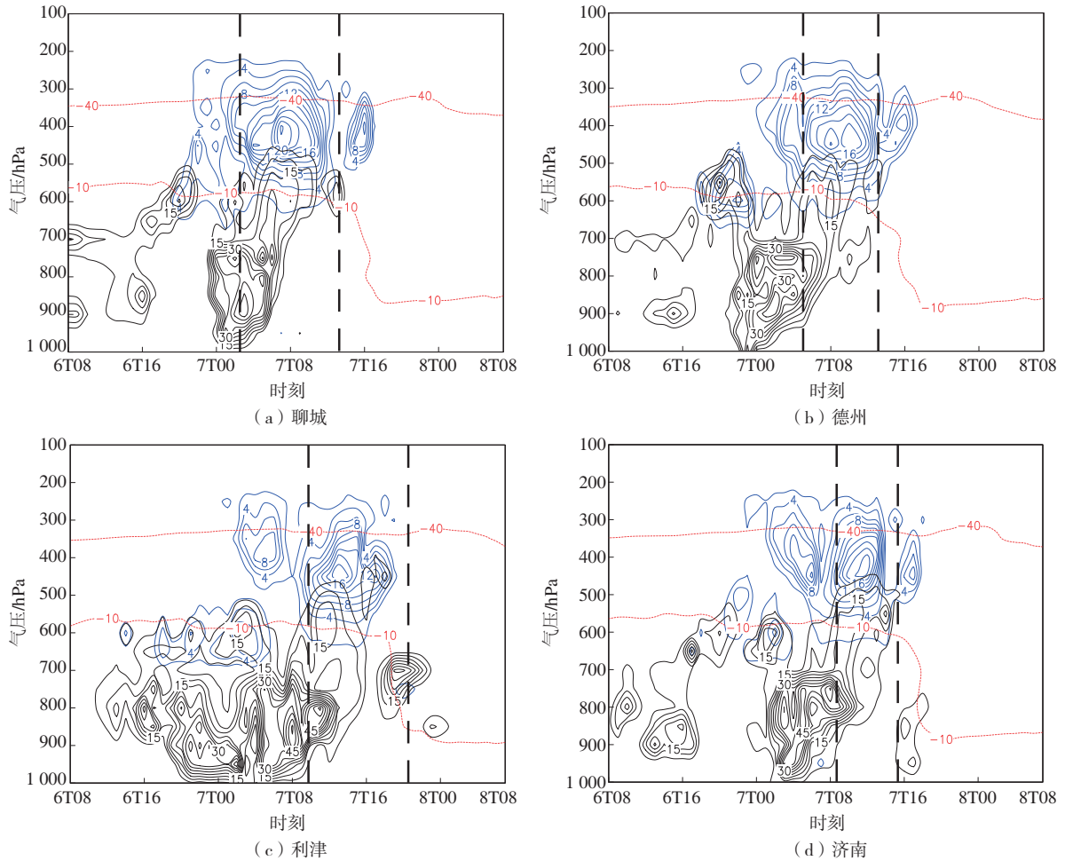
蓝色等值线—冰相粒子, 单位: 10^{-5} \text{ kg} \cdot \text{kg}^{-1} ; 黑色等值线—液态水粒子, 单位: 10^{-5} \text{ kg} \cdot \text{kg}^{-1} ; 红色虚等值线—温度, 单位: °C; 黑色虚线区域—降雪时段。
