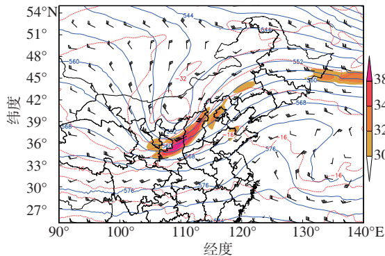
(a) 500 hPa 位势高度场
