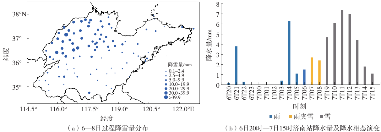
图1 山东 2021 年 11 月 6—8 日降雪过程气象要素分布
