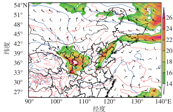
(b) 700 hPa 位势高度场
