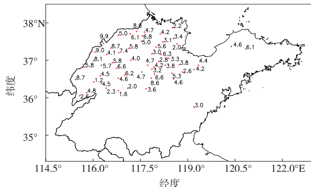
(a) 过程平均雪水比分布
