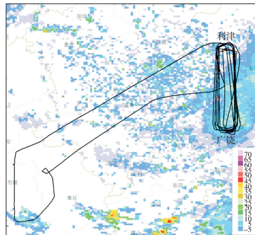
色阶—2019年11月17日15:04滨州雷达组合反射率因子,单位为dBZ。
