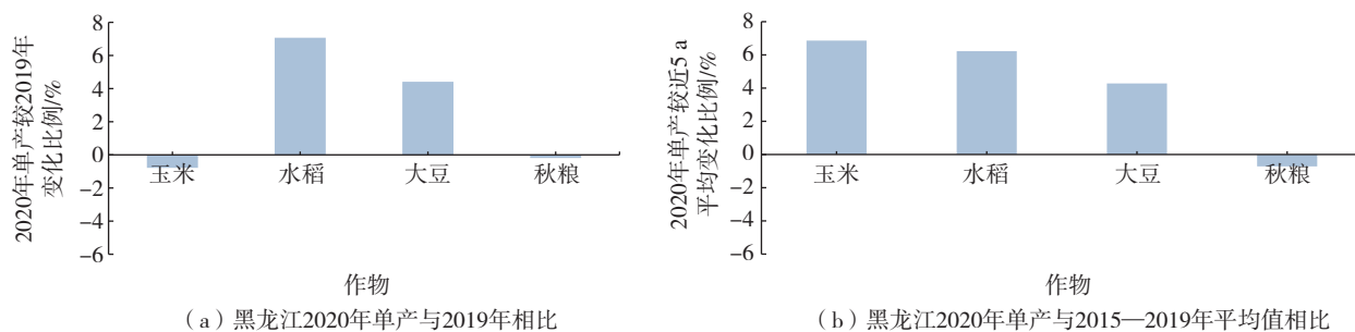
图7 黑龙江2020年单产与2019年、2015—2019年平均值相比
