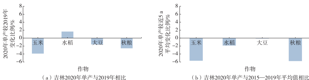
图 6 吉林 2020 年单产与 2019 年、2015—2019 年平均值相比
