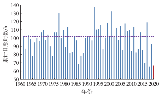
图5 吉林1961—2020年历年8月26日—9月8日 累计日照时数
